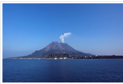
櫻島火山
